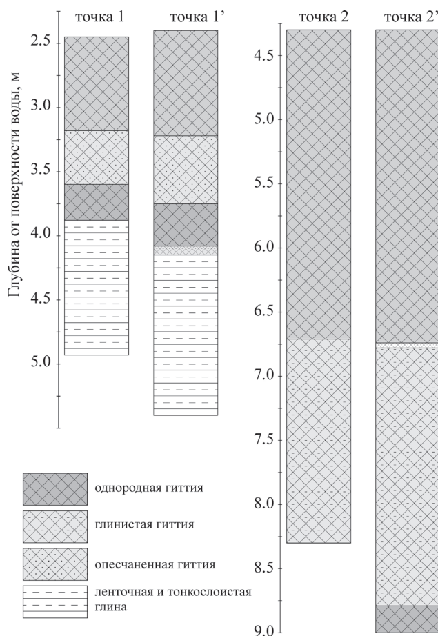
Рис. 3. Стратиграфия разрезов.
